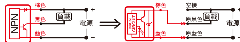
兩線式替換NPN型接法(原棕色線空接)
