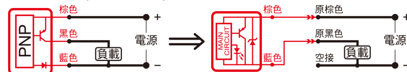
兩線式替換PNP型接法(原藍色線空接)
