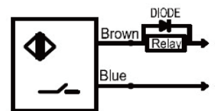
接線圖： Relay Load Sink(NPN) Wiring diagram
